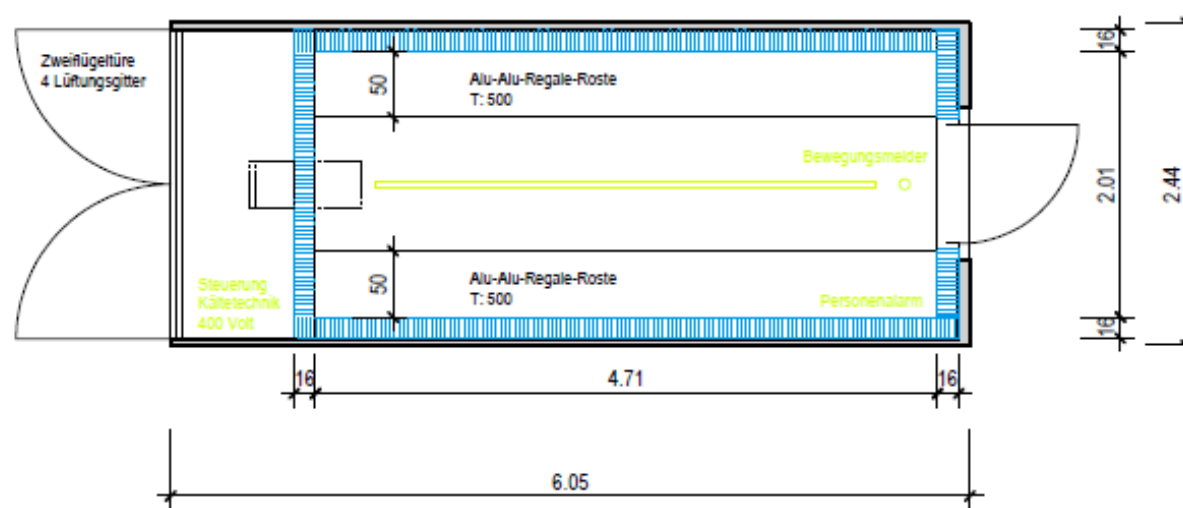
Grundriss
